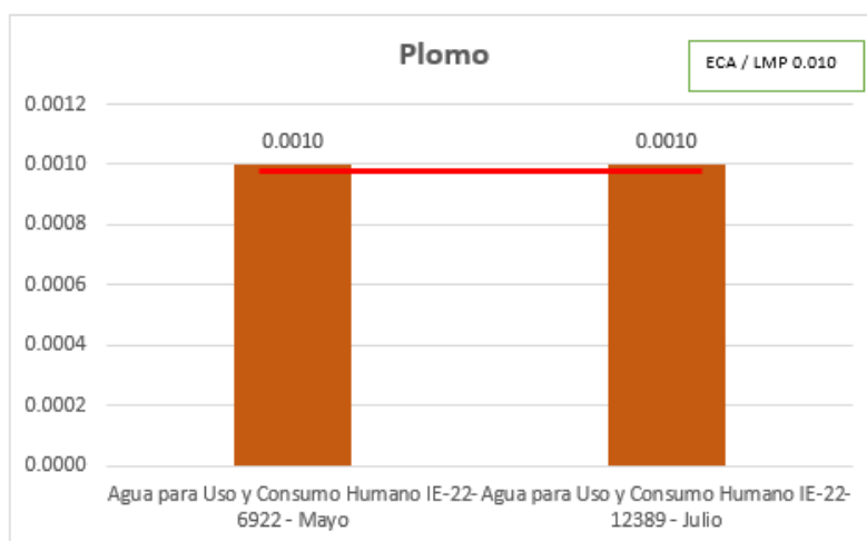
Figura 28: Comportamiento de Plomo de la estación AG-GR
