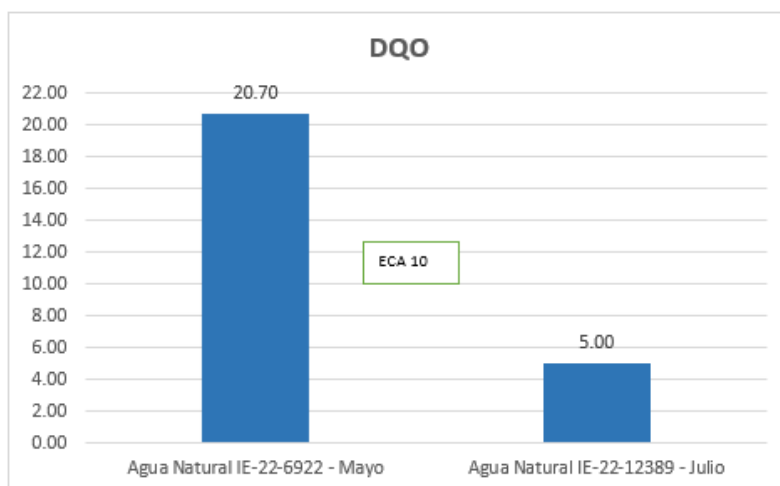
Figura 16: Comportamiento del DQO de la estación AG-Captación
