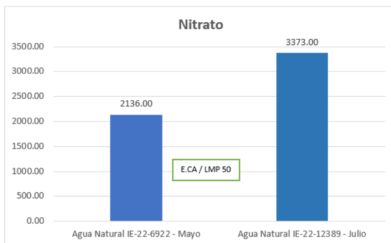
Figura 17: Comportamiento de Nitrato de la estación AG-Captación
