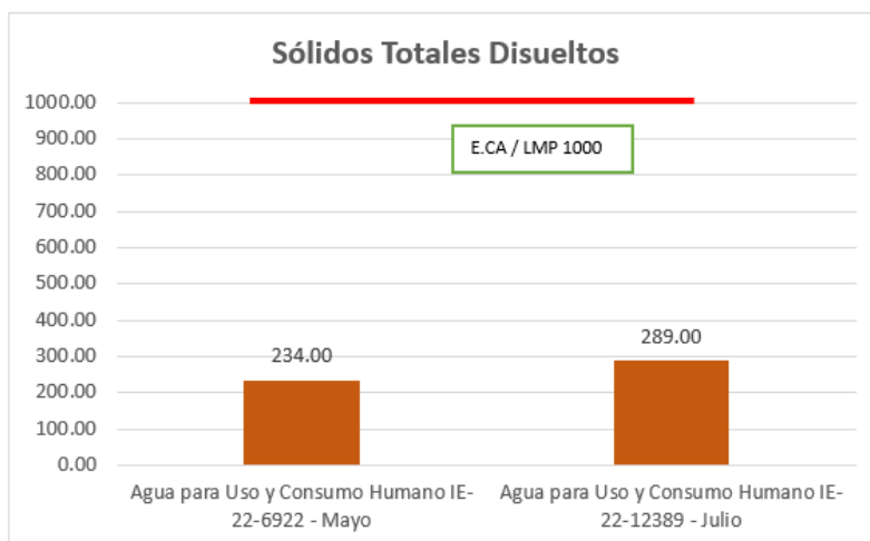
Figura 20: Comportamiento de Sólidos Totales Disueltos de la estación AG-GR
