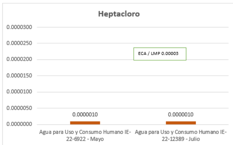
Figura 30: Comportamiento de Heptacloro de la estación AG-GR
