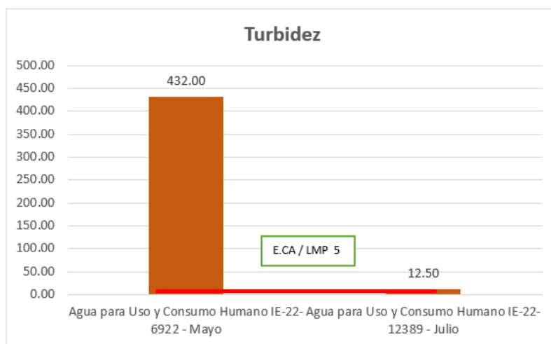
Figura 8: Comportamiento de Turbidez de la estación AG-GR
