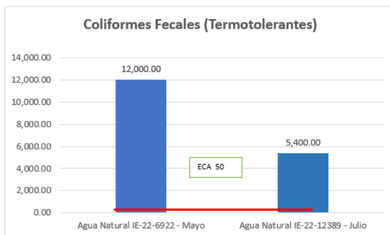
Figura 33: Comportamiento de Coliformes Fecales de la estación AG-Captación
