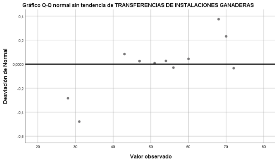
Figura 26. Gráfico Q-Q.
