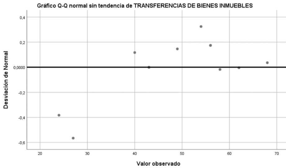
Figura 18. Gráfico Q-Q.
