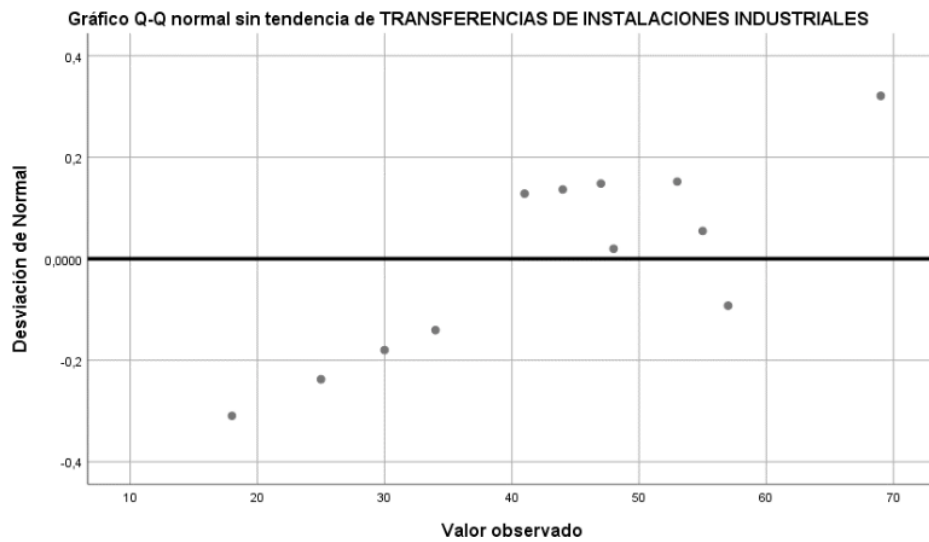
Figura 22. Gráfico Q-Q.
