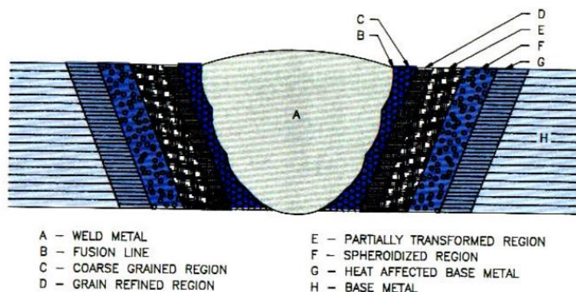
Figura 2: Esquema de la Microestructura de una Soldadura de un acero micro aleado.
