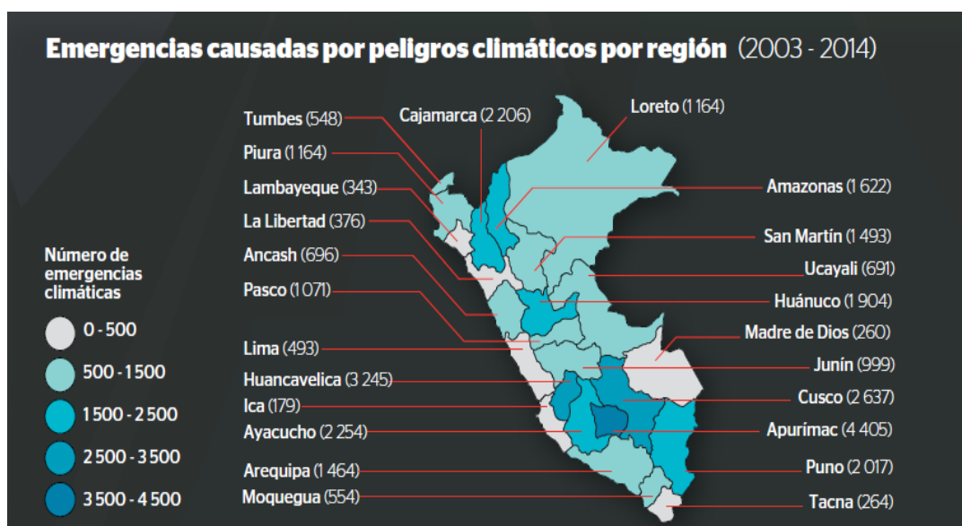
Figura 1. Emergencias por cambios climáticos por región (2003-2014)
