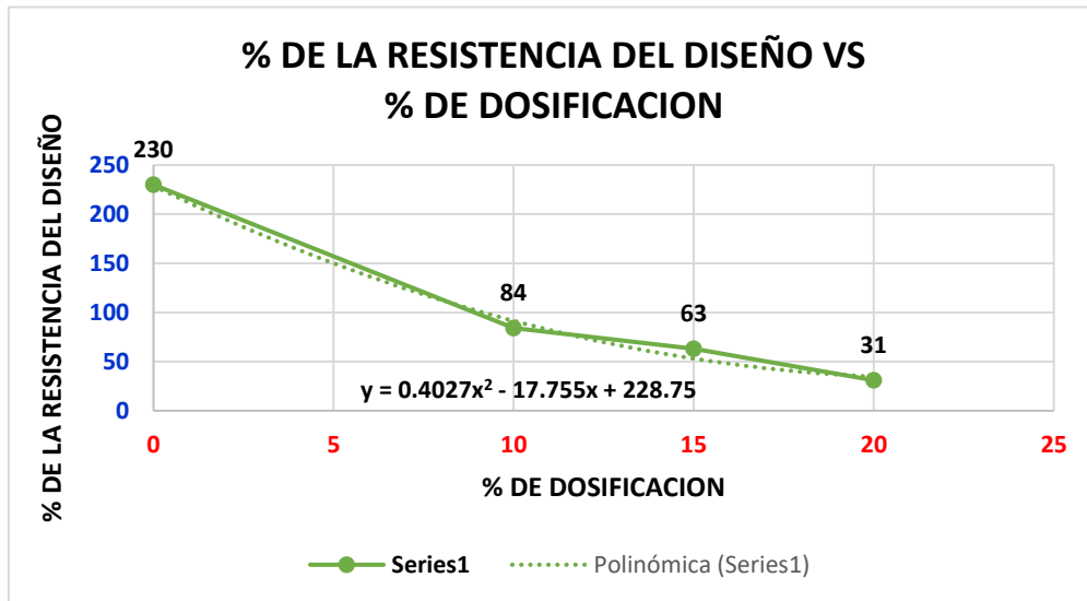
GRÁFICO N 6: Porcentaje de la resistencia del diseño vs Porcentaje de dosificación.
