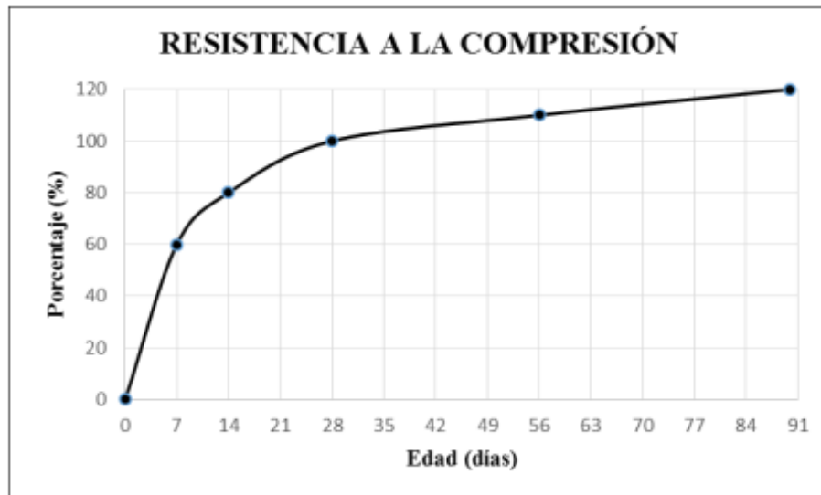
Figura 2: Curva de Resistencia a la Compresión en Función del Tiempo.
