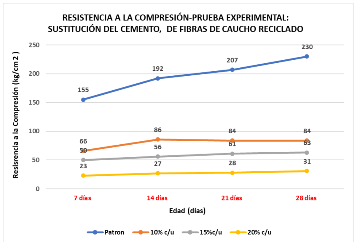
GRÁFICO N 5: Comportamiento de la Prueba Patrón y Prueba Experimental en el Tiempo
