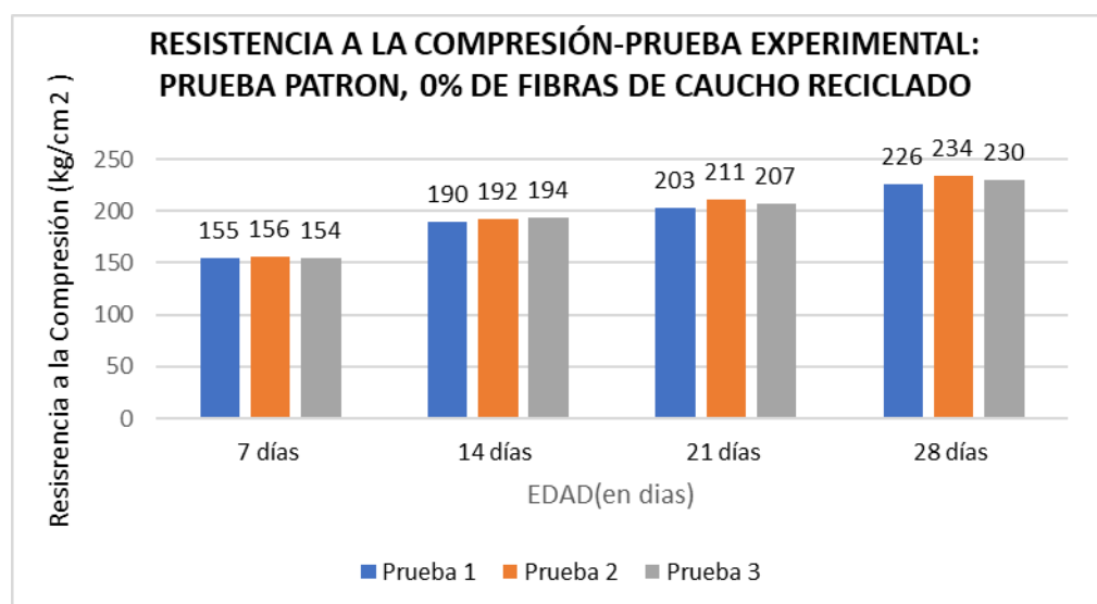
GRÁFICO N° 1: Resistencia a la Compresión-Prueba Patrón
