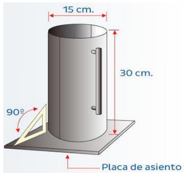
Figura 4: Molde para las Probetas
